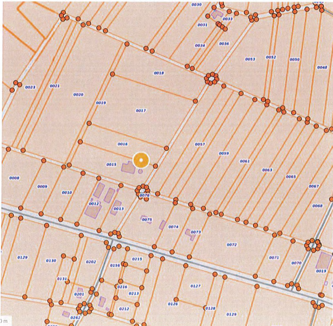
Extrait cadastral
